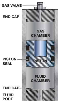
PISTON TYPE
